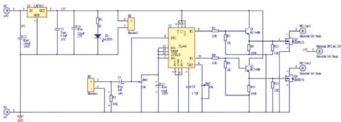
Rys. 1. Schemat płytki PCB głośnika plazmowego
